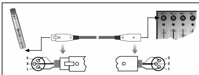
Fig. 4 : Branchement sur entrée symétrique avec alimentation fantôme.
